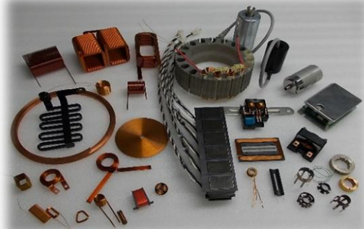
↑(各種コイル)
